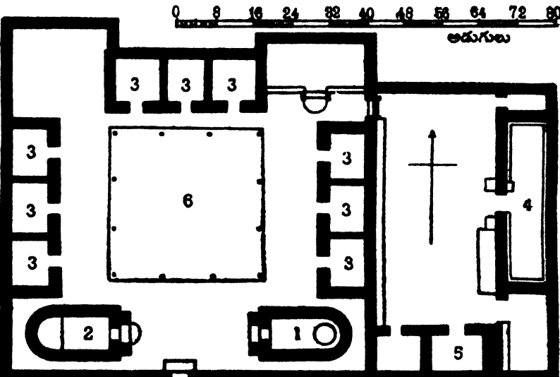
చిత్రము 6. బౌద్ధ విహారము : అందలి భాగములు 1. స్తూప చైత్యము, 2. బద్ధ చైత్యము, 3. బౌద్ధ లిఖిత మందిరములు, 4. భోజనశాల, 5. పాకశాల, 6. మండపము.
